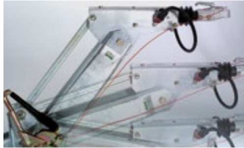
Höhenverstellbare Zugdeichsel (Kugelpfropfkupplung und DIN-Zugöse nicht inklusive)
